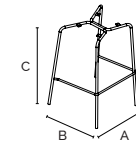
12 xylo - telaio sgabello h.750 d.16 senza tappi xylo - stool frames h.750 d.16 without caps
