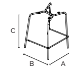
11 xylo - telaio sgabello h.650 d.16 senza tappi xylo - stool frames h.650 d.16 without caps
