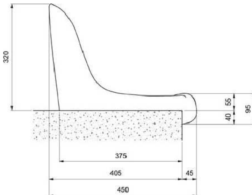
מידות המושב
